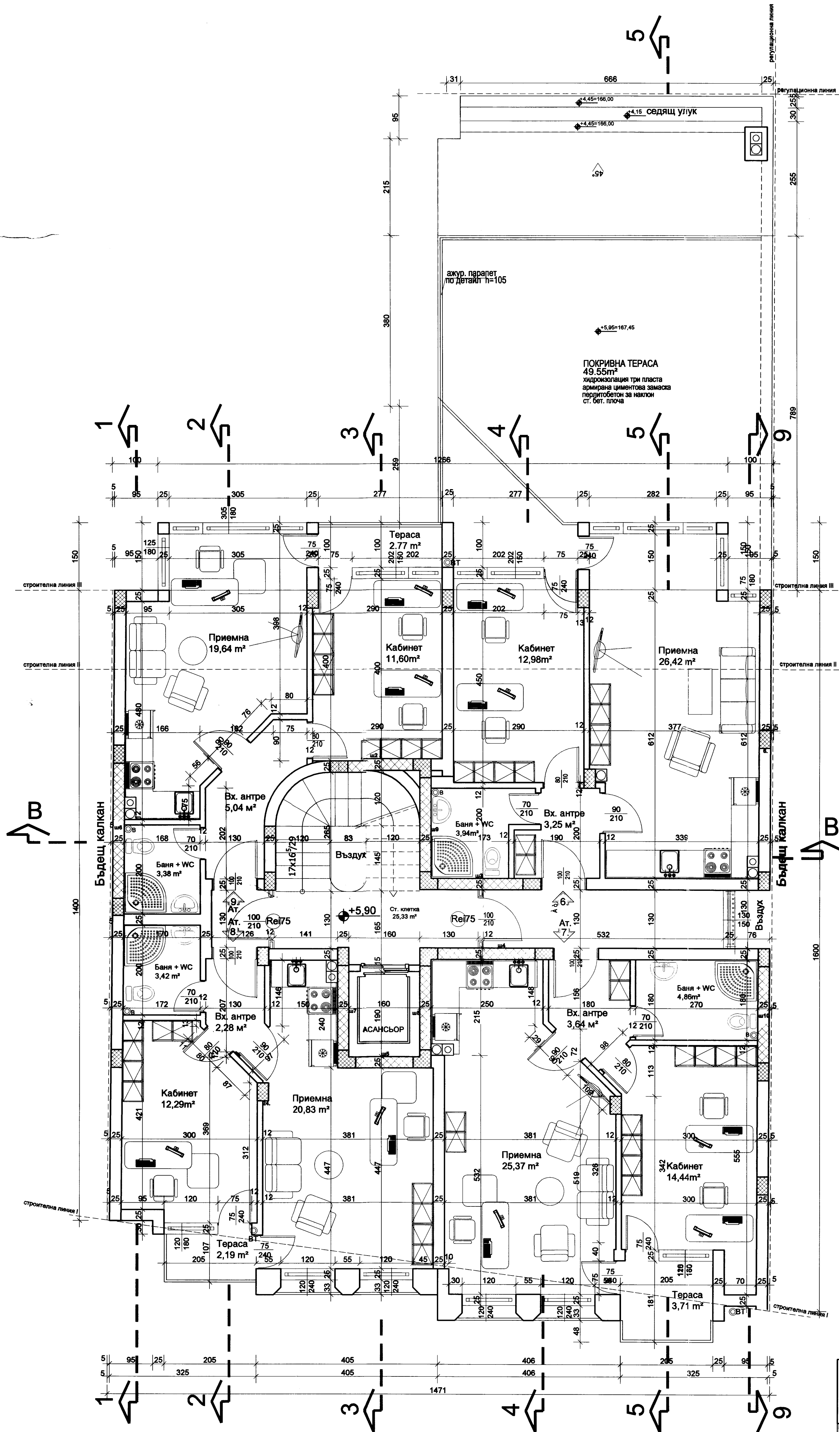
РАЗПРЕДЕЛЕНИЕ - ЕТАЖ III КОТА +5.90 М 1:50
