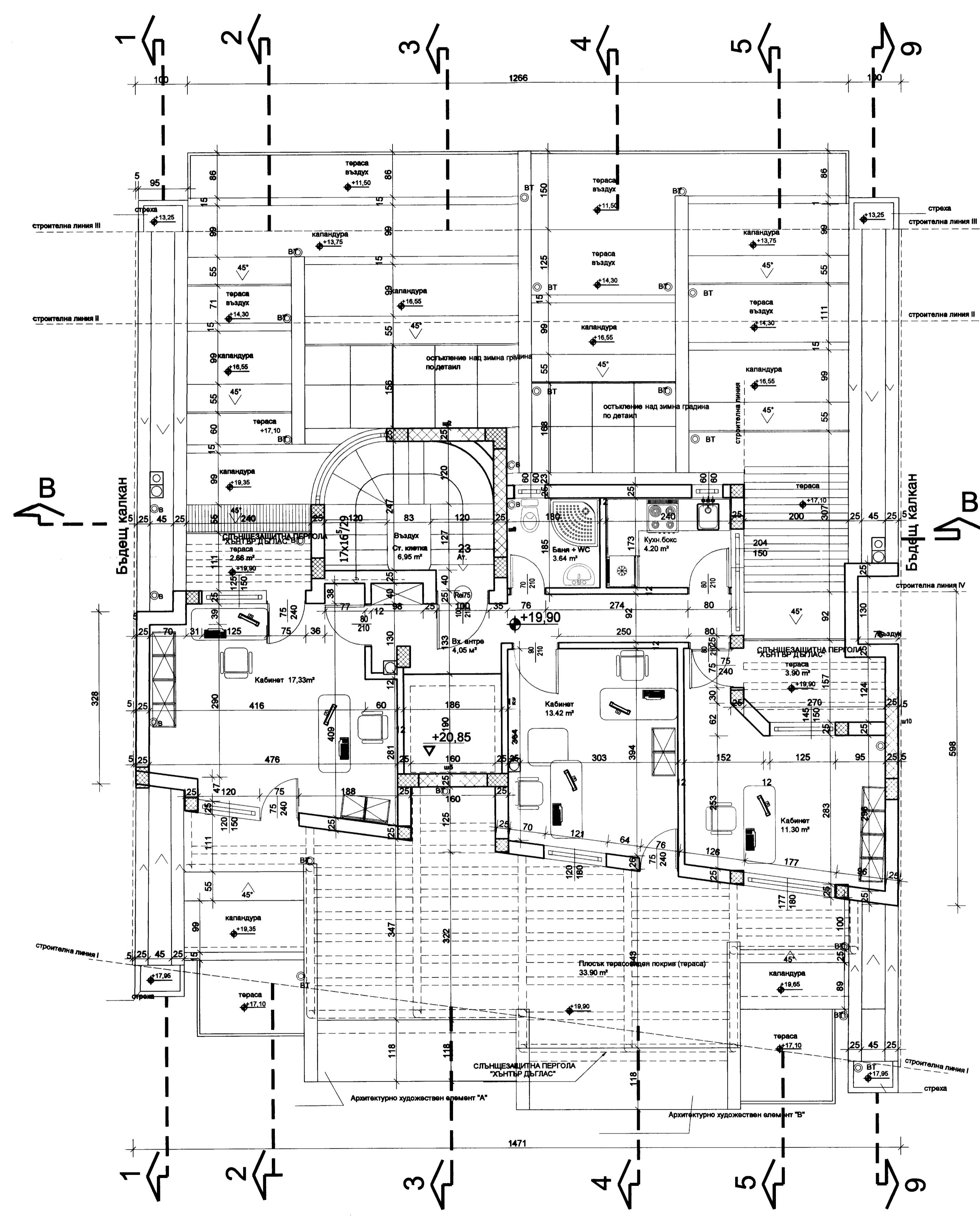
РАЗПРЕДЕЛЕНИЕ - МАНСАРДЕН ЕТАЖ II НИВО КОТА +19.90 М 1:50
