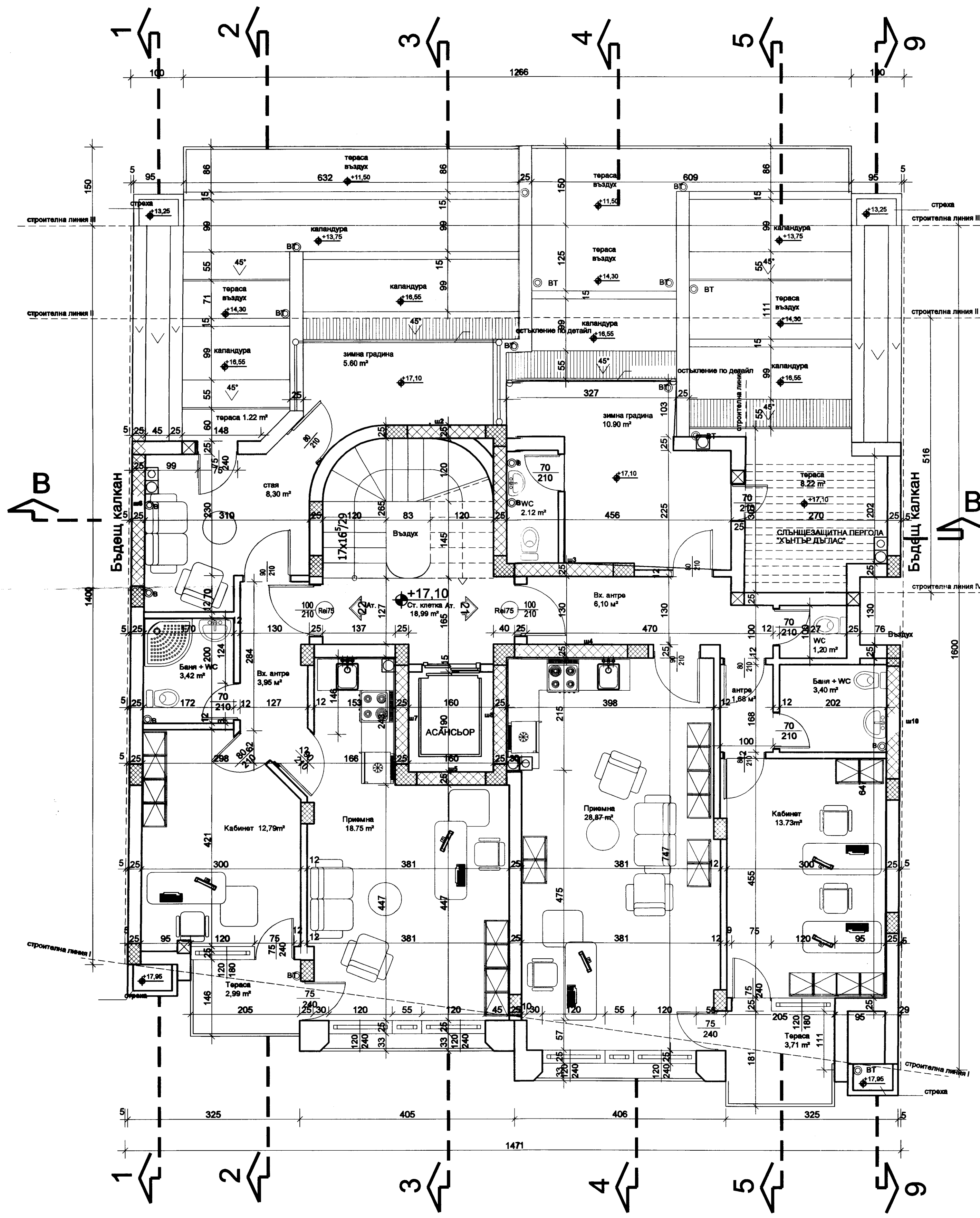
РАЗПРЕДЕЛЕНИЕ - МАНСАРДЕН ЕТАЖ I НИВО КОТА +17.10 М 1:50
